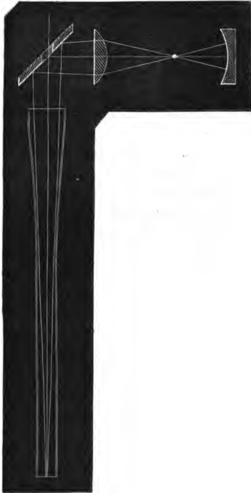
Fig. 1. — Théorie de l'endoscope.
